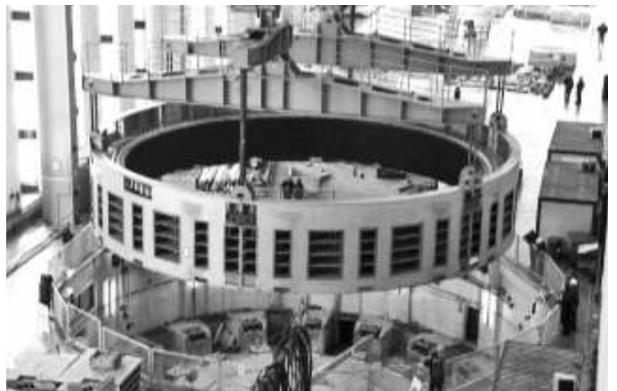
Радови на монтажи статора
